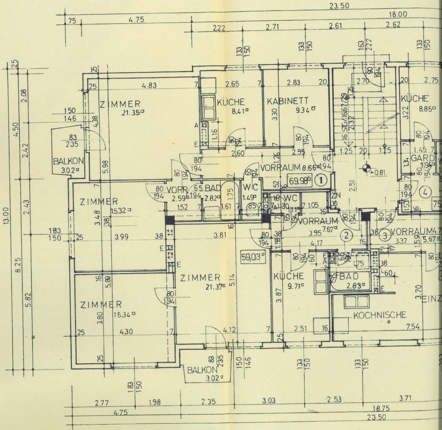
ERDGESCHOSS 1:100
