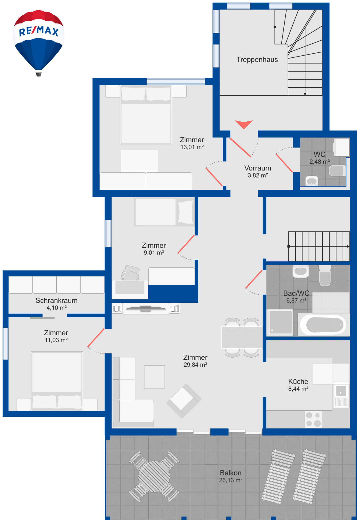
Obergeschoss
