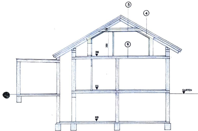
SNITT A-B
