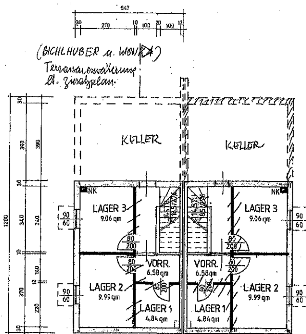
KELLER
