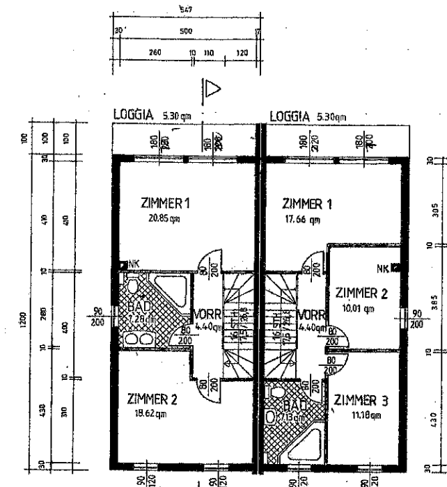
OBERGESCHOSS
