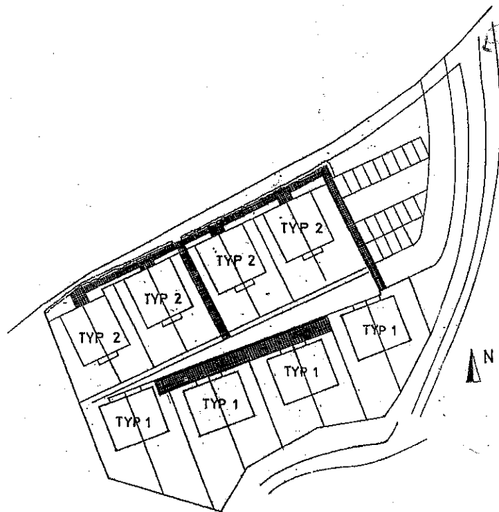
LAGEPLAN
