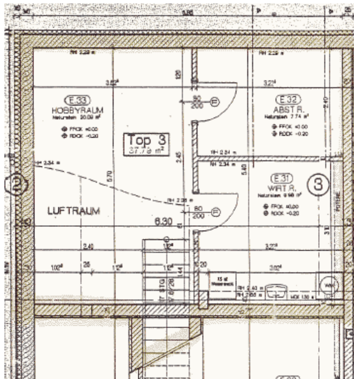
Untergeschoß
