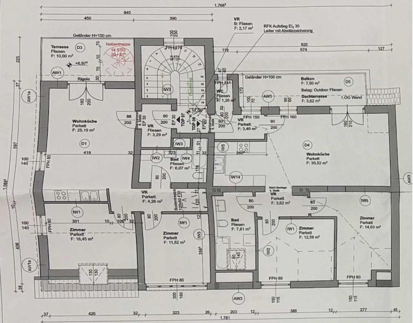
DACHGESCHOSS 1:100
