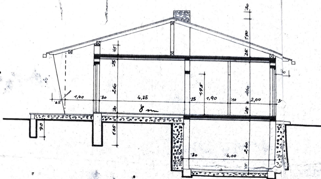
SCHNITT:
