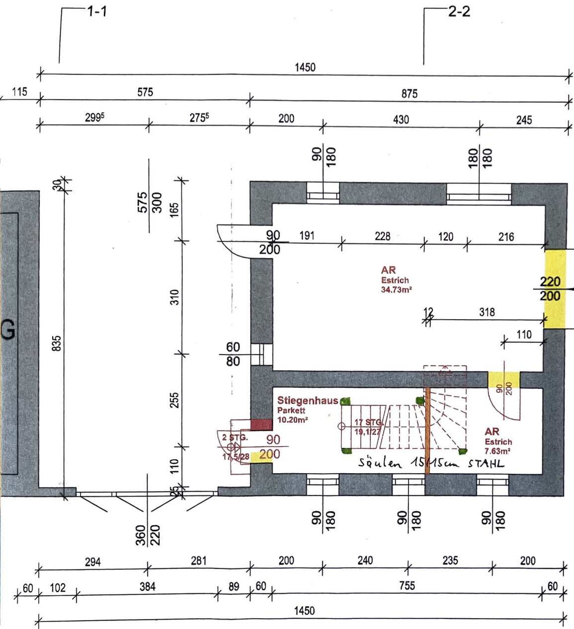
GRUNDRISS ERDGESCHOSS 1:100
